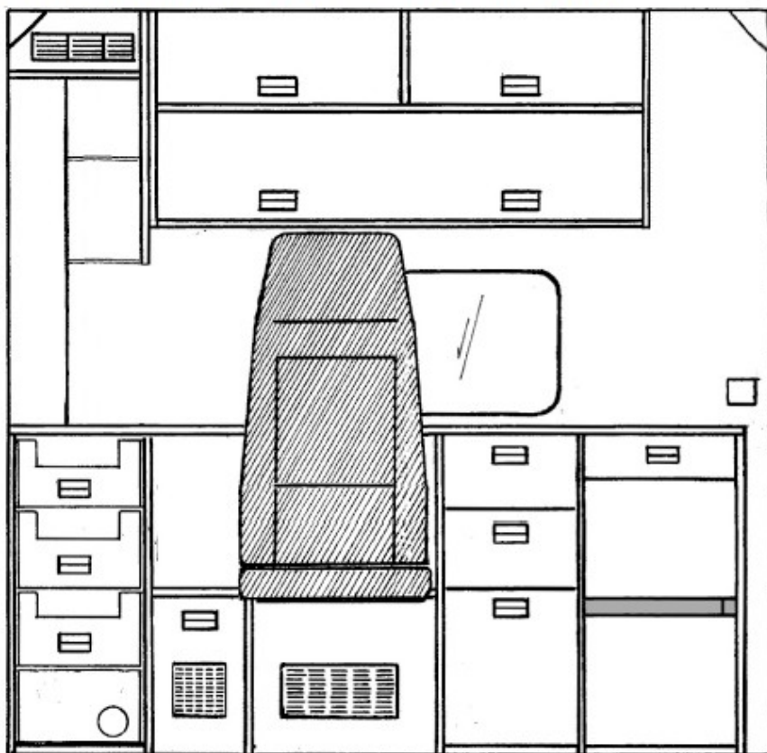
Schema nábytkové zástavby vozidla typ C, dělicí přepážka
