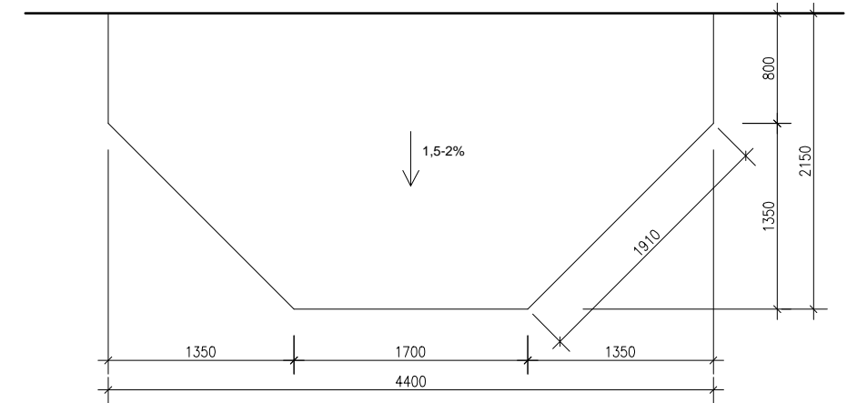
ŘEZ BALKÓNOVOU DESKOU
