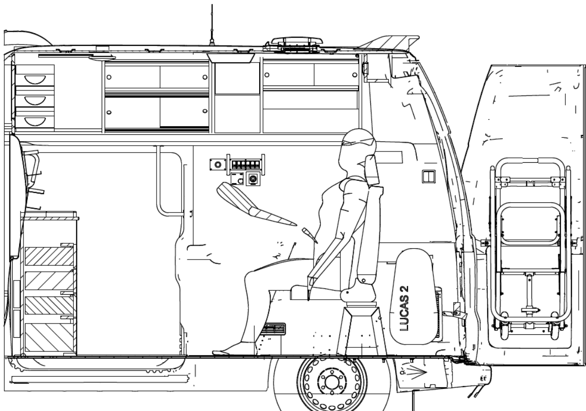
Příloha: Příklad uspořádání zástavby ambulantního prostoru na průřezech
