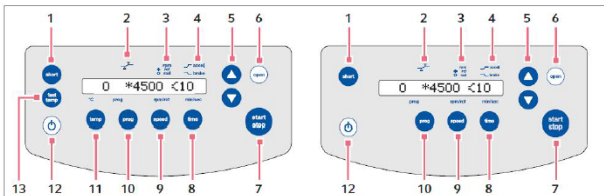
Obr. 5-1: Ovládací prvky centrifug 5804 R/5810 R a centrifug 5804/5810
