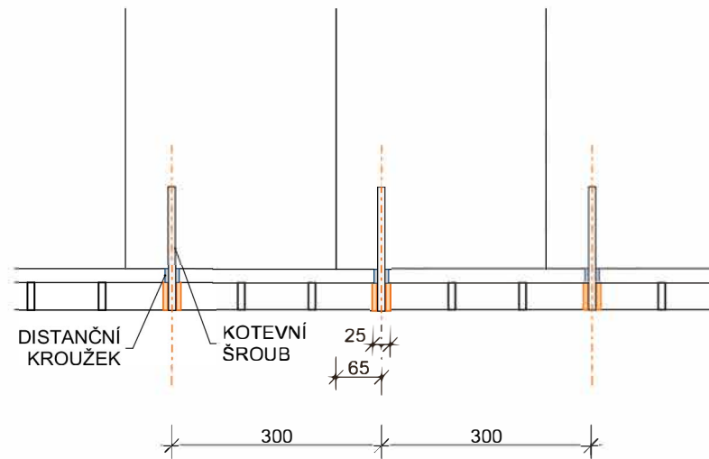
DETAIL KOTVENÍ ZÁBRADLÍ - PŮDORYS:
