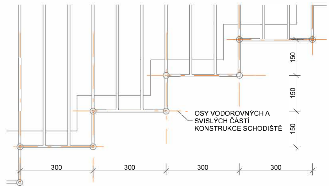
DETAIL KOTVENÍ ZÁBRADLÍ - POHLED BOČNÍ:
