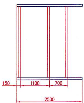
SI - Systém lehký poleťový/alternativně UZ 300kg/m 2
