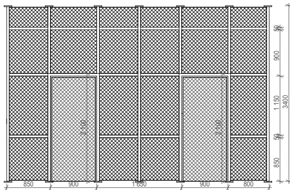
POHLED A4-OCELOVÁ STĚNA S PLETIVEM MÍSTNOST D.01.027 , D.01.029 , D.01.030
