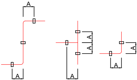
ZPŮSOB UCHYCENÍ POTRUBÍ A = max 500 mm
