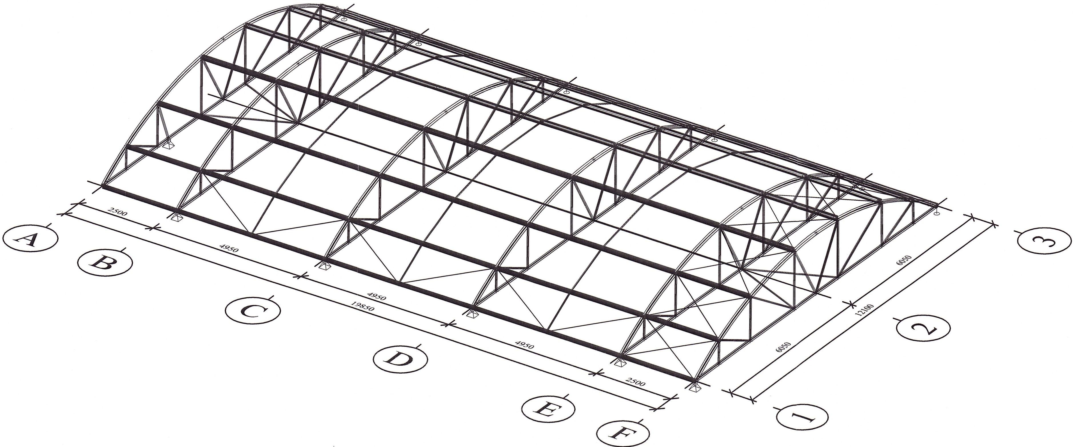
IZOMETRICKÝ POHLED
