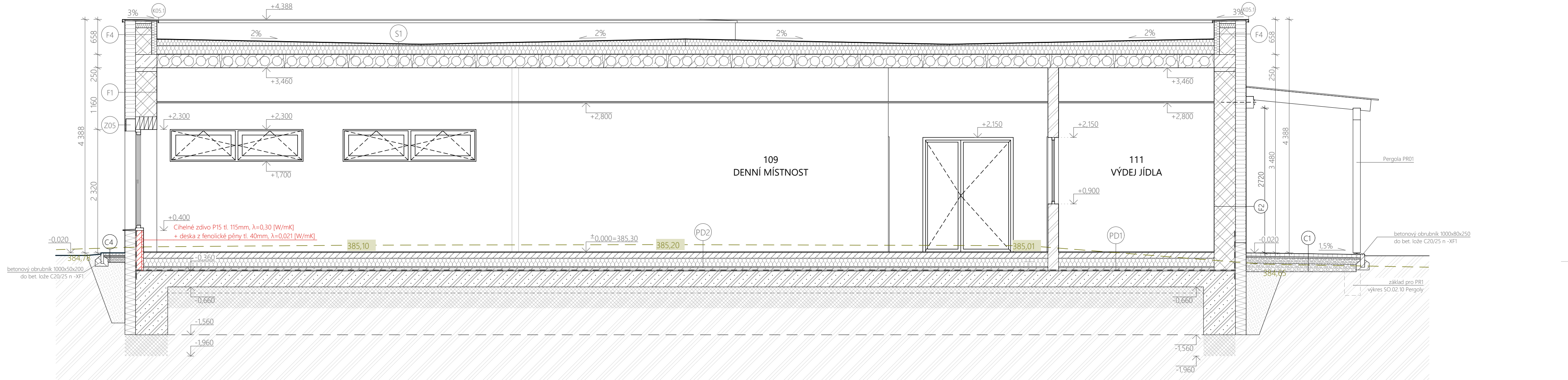
ŘEZ B-B':
