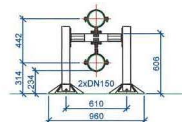
K5 KLUZNÉ ULOŽENÍ
