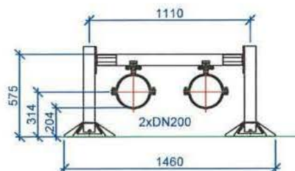
K1 KLUZNÉ ULOŽENÍ
