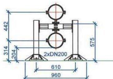
K4 KLUZNÉ ULOŽENÍ
