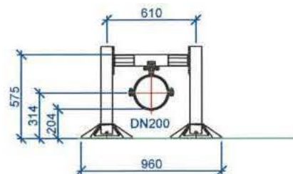
K3 KLUZNÉ ULOŽENÍ
