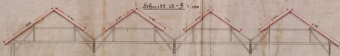
Obr. 4: Plán na rekonstrukci střešní krytiny „Fuhrwerk Depot I a II“v Josefově z r. 1914. Zdroj: VHÚ Praha
