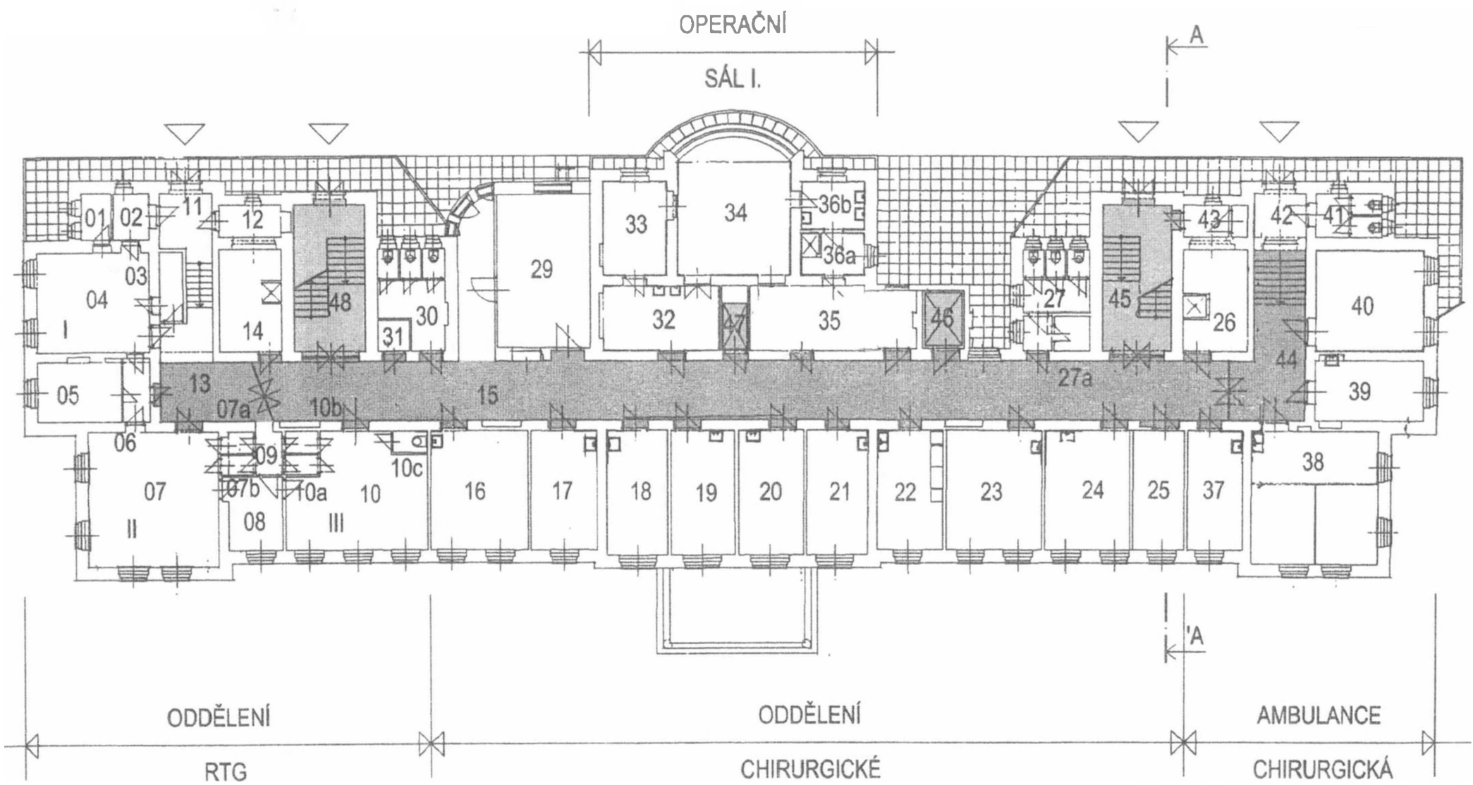
Hl. budova - 1.NP (1:250)
