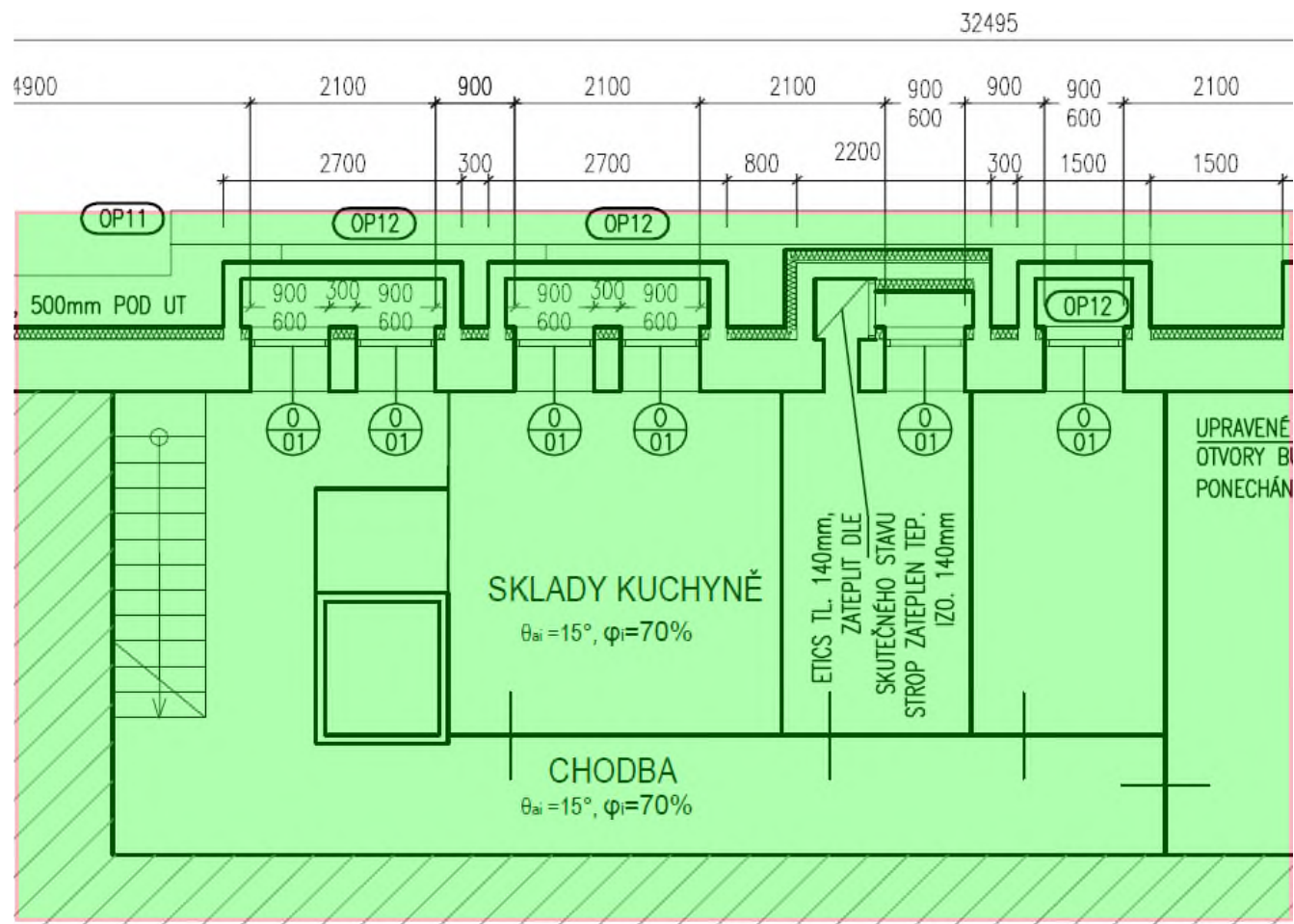
1 podzemní podlaží gastro provozu
