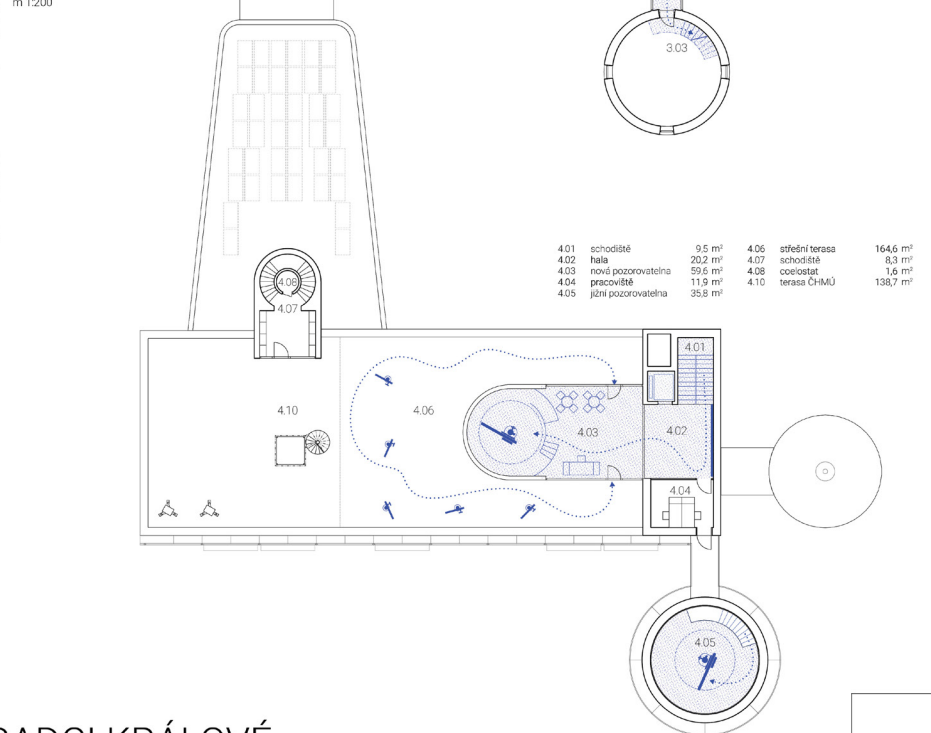
půdorys 4.np m 1:200
