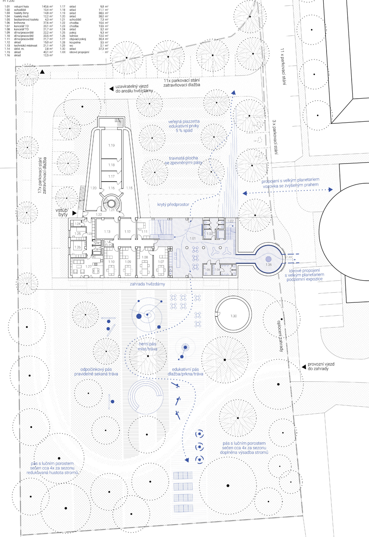
půdorys 1.np / vstupní podlaží m 1:200
