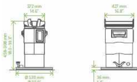
Stacionární sloupek, verze B
