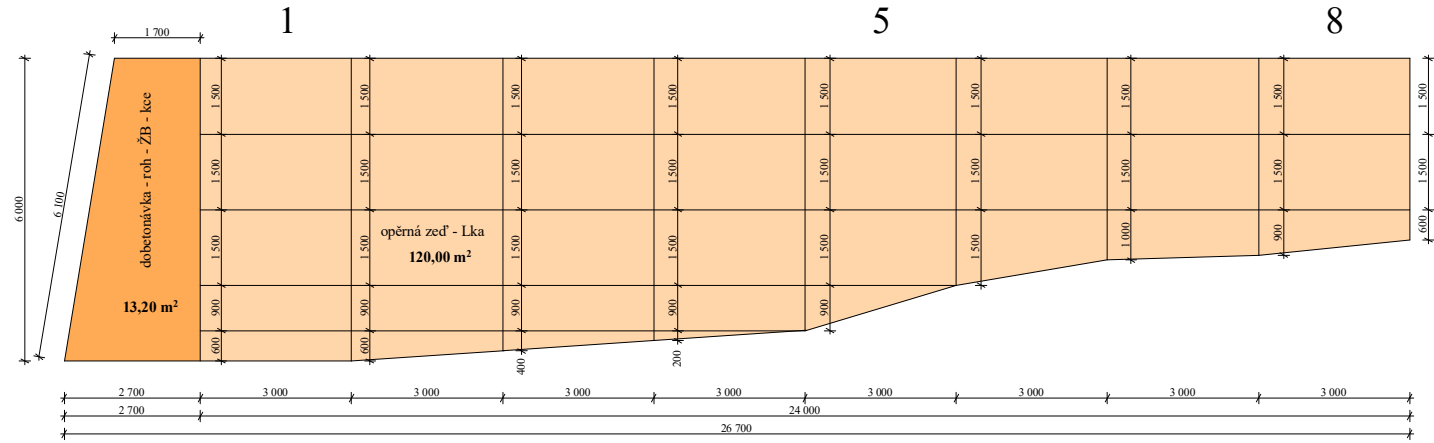
ZOO DK - OPRAVA - opěrná zeď - východní pohled
